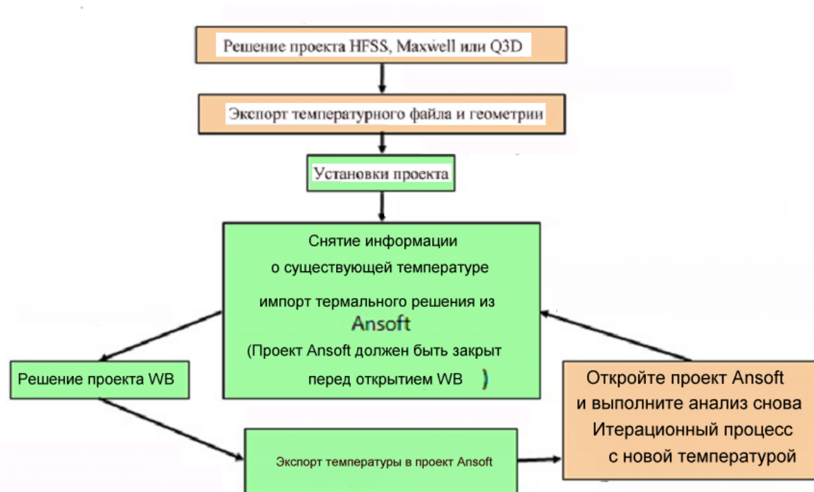
Рис. 9.10. Расчет температурных характеристик с помощью Re-solving After ANSYS Thermal Link Feedback
