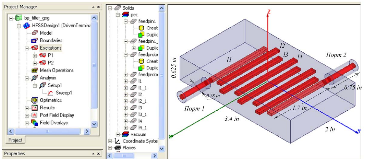
Рис. 8.1. Вид фильтра в интерфейсе HFSS-13
