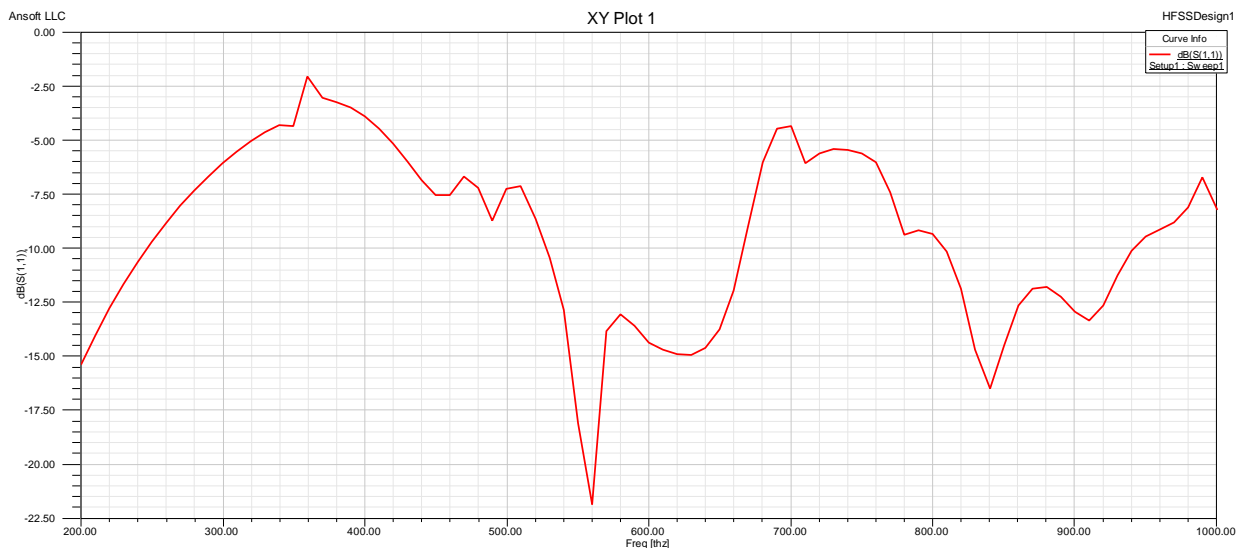
Рис. 15.46. Частотная характеристика S_{11} по каждому порту, внедренному в КК (8 портов)
