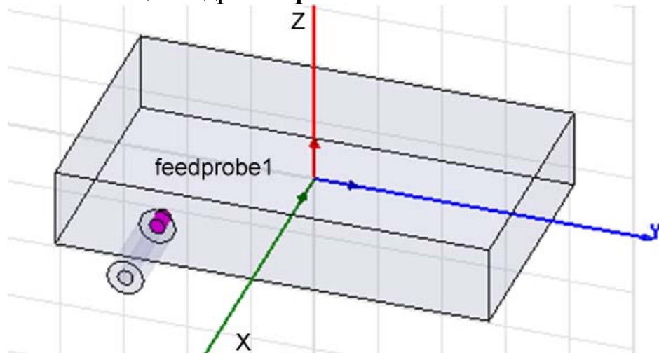
Рис. 8.11. Штырек связи с фильтром
