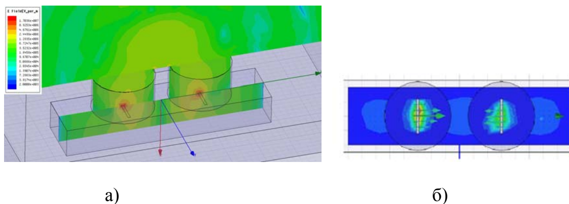
Рис.15.22. Излучение из КТ (а) в момент времени, когда в щелях связи максимальное электрическое поле (б)
