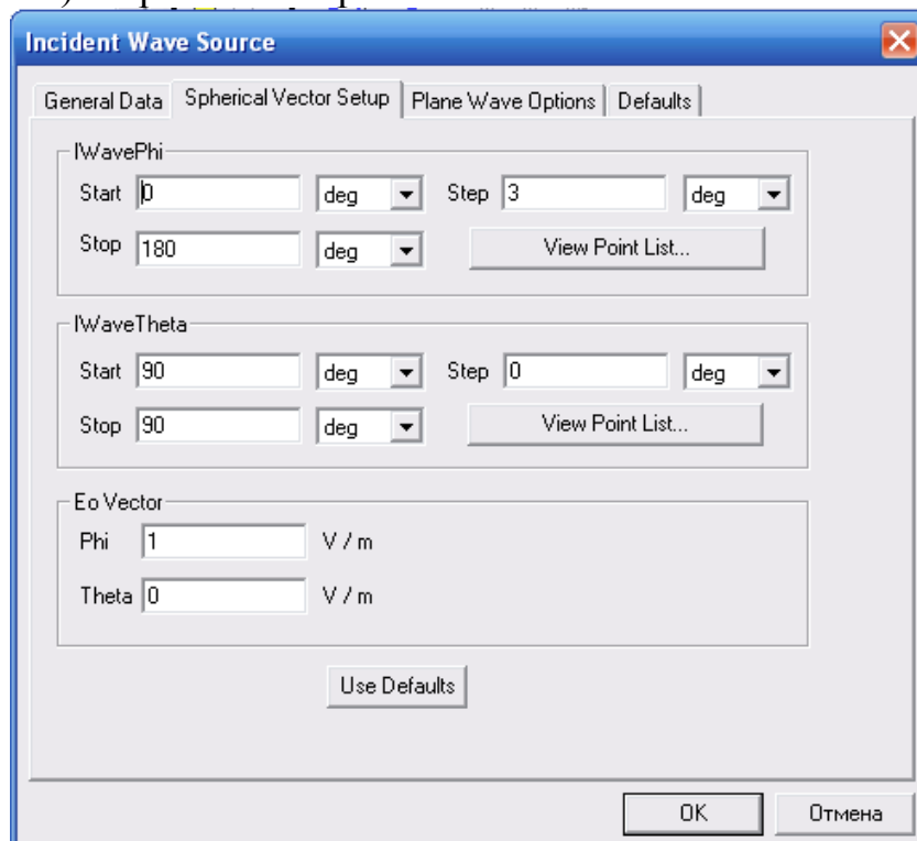
Рис. 6.2. Параметры плоской волны с установками для расчета моноимпульсного РСР
