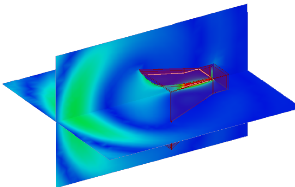
Рис. 14.29. Распространение поля в двух перпендикулярных плоскостях
