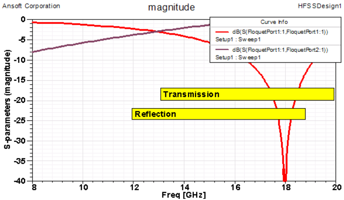
Рис. 5.16. Частотные характеристики модулей коэффициентов отражения и передачи ЧСП по основной волне
