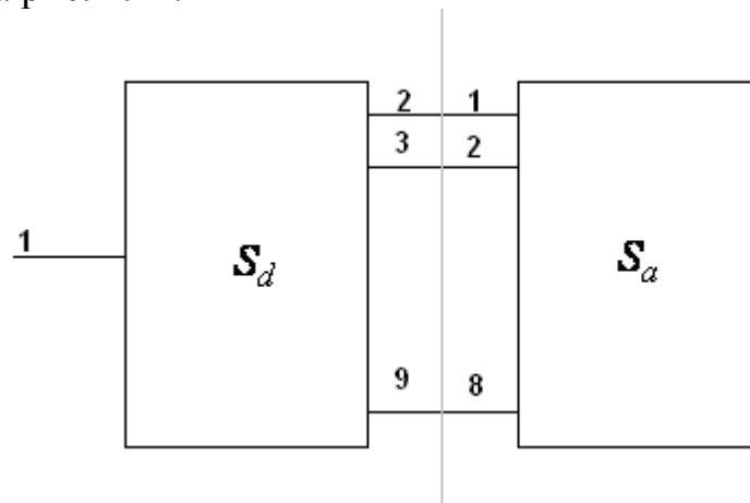
Рис. 4.21. Каскадное соединение МДМ и решетки
