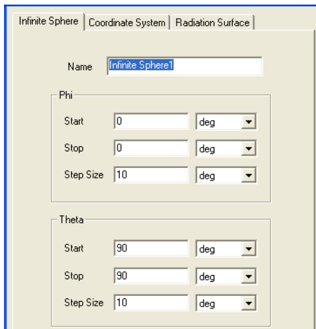
Рис. 7.13. График установки данных расчета дальнего поля. Фактически один угол \phi и один угол \Theta
