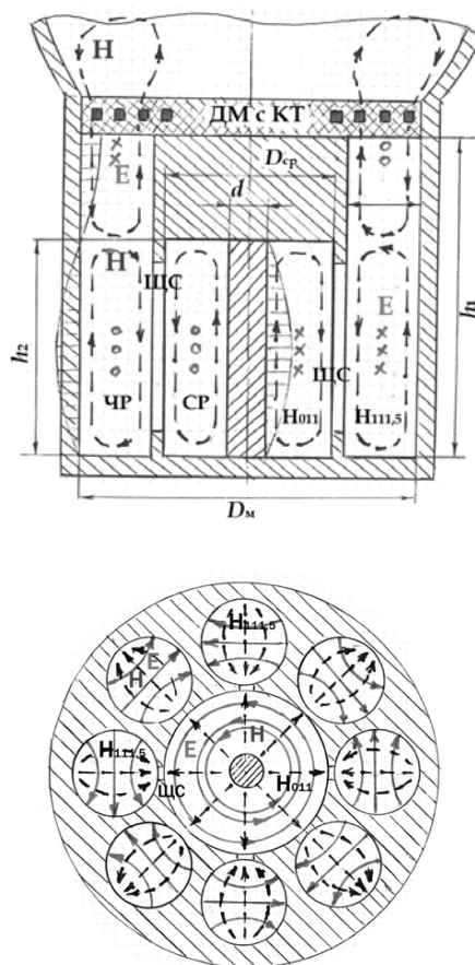
Рис. 15.30. Излучатель с коаксиальным стабилизирующим резонатором.
