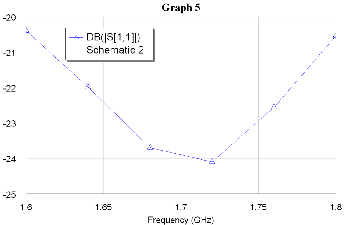
Рис. 4.20. Частотная зависимость коэффициента отражения МДМ по входу 1
