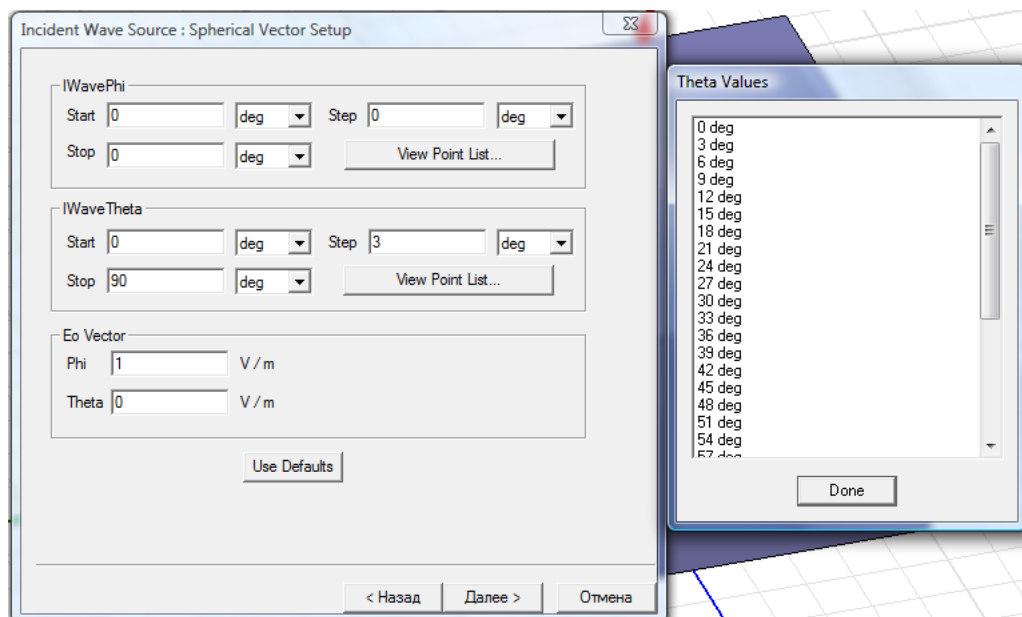
Рис. 6.12. Параметры падающей плоской волны
