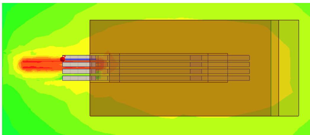
Рис. 11.13. Рассчитанное поле E в сечении линий передачи, при возбуждении 1-го порта
