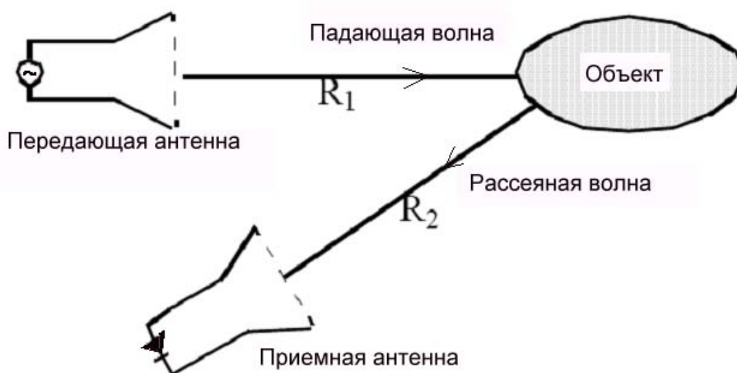
Рис. 6.1. Схема бистатической радиолокации
